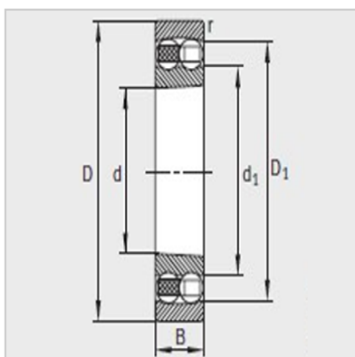
圆锥孔 K = 锥度1:12
