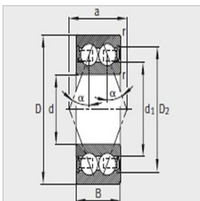
38..-B-2RSR、30..-B-2RSR、 32..-B-2RSR、33..-B-2RSR \alpha = 25^\circ
