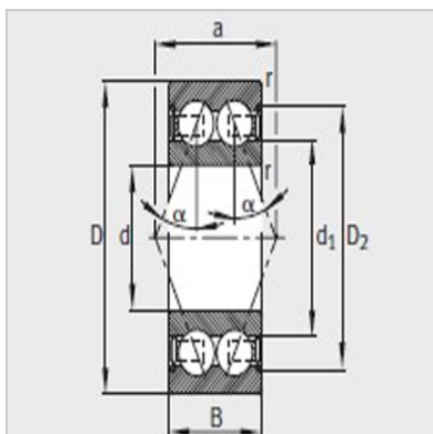
38..-B-2Z、30..-B-2Z、32..-B-2Z、33..-B-2Z \alpha = 25^\circ
