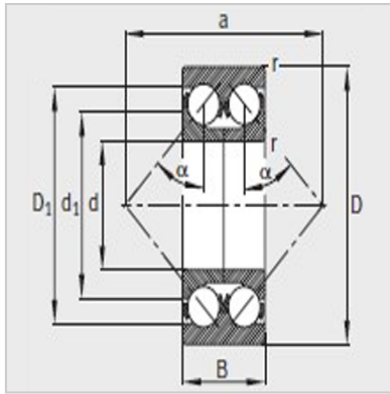
33..-DA 双内圈 \alpha = 45^\circ
