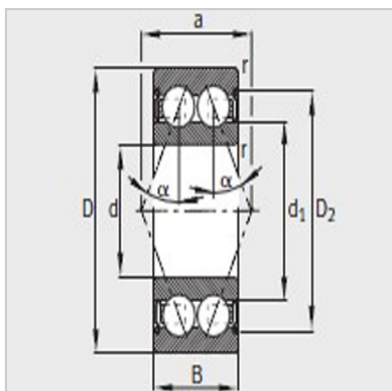
38..-B-2Z、32..-B-2Z \alpha = 25^\circ
