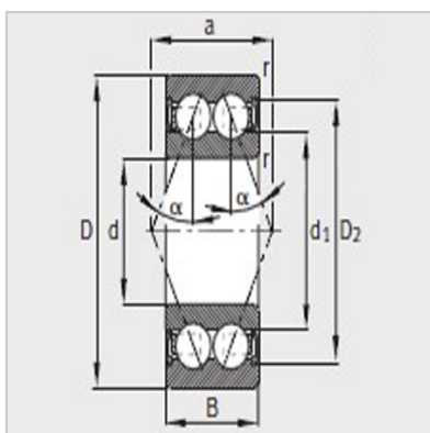
38..-B-2RSR \alpha = 25^\circ
