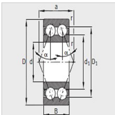
38..-B、32..-B \alpha = 25^\circ
