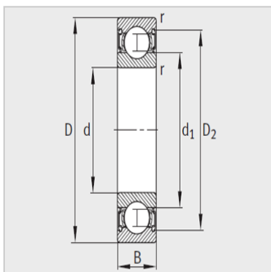
密封2RSR
