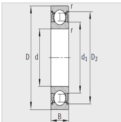
防尘盖2Z
